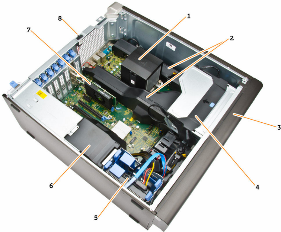
Ilustración 2. Vista interior del equipo T5810
